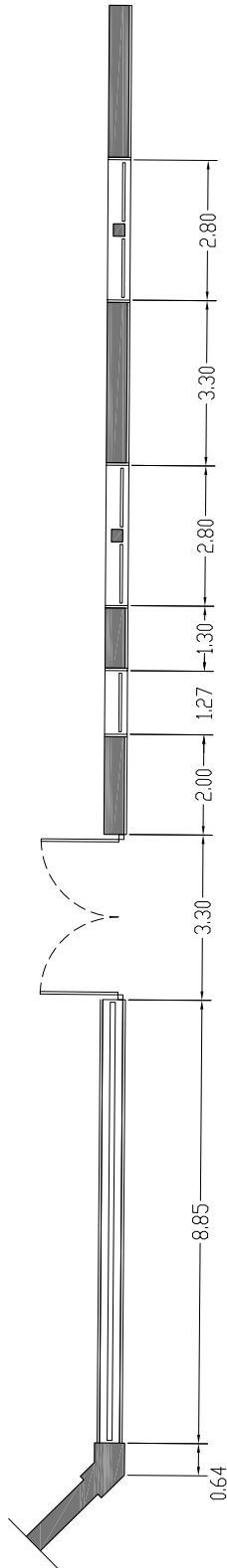
PLANTA DE REFERÈNCIA DE L'ESTAT ACTUAL DEL MUR EXTERIOR. FRONT CARRER VILADOMAT
